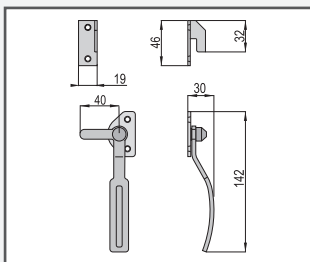
Zapiralna ročica iz pocinkanega in kromiranega železa.
