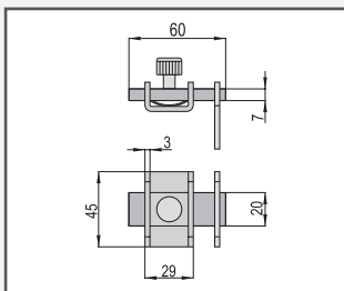
Zapiralo iz pocinkanega železa za privarit.
