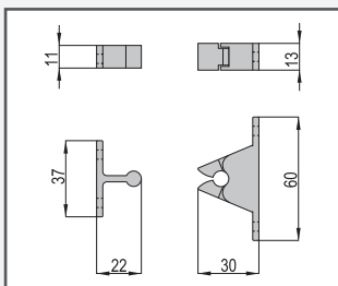
Zapiralo v bronirani obdelavi.
