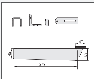
Samozapiralo za vrata v črni barvi. Možna nastavev hitrosti zapiranja in končnega udarca.
