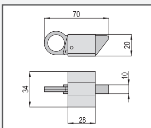
Zaskočnik iz železa.
