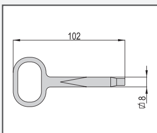
Ključ za zapiralo CS8.
