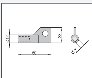
Ključ za zapiralo T7.
